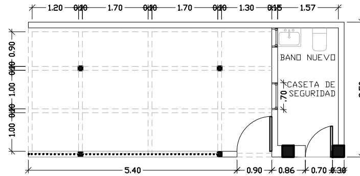
2 A-1 PLANTA DIMENSIONADA CUBIERTA EXTERIOR Y CASETA ESC. 1:150
