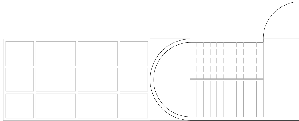
1 A-1 PLANTA DE TECHO CUBIERTA EXTERIOR Y CASETA ESC. 1:150
